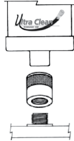
Накидной адаптер Модель UC-AD105 (1"- 12 UNF) Модель UC-AD106 (1 1/2"- 16 OOH)
