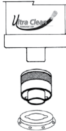
Штыковой адаптер Модель UC-AD104
